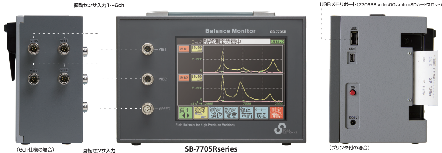
USB mini-Bタイプコネクタ
