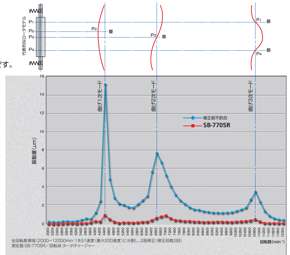
振動実測グラフ
